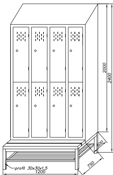
No.67 Szafa 2x4 z ławką
