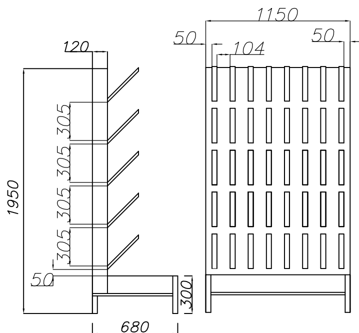
No.87 Suszarka do butów
