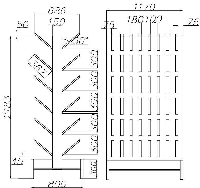
No.88 Suszarka do butów
