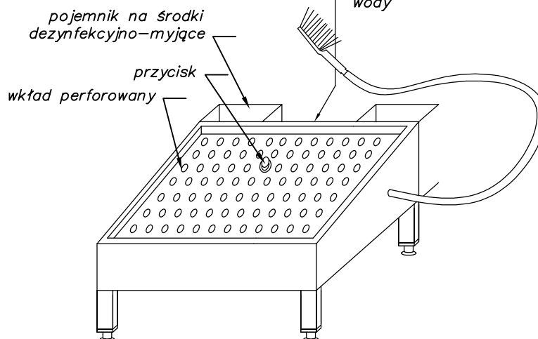
No.84 Myjka butów
