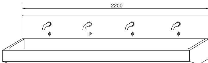
No.50 umywalka 4 stanowiskowa
