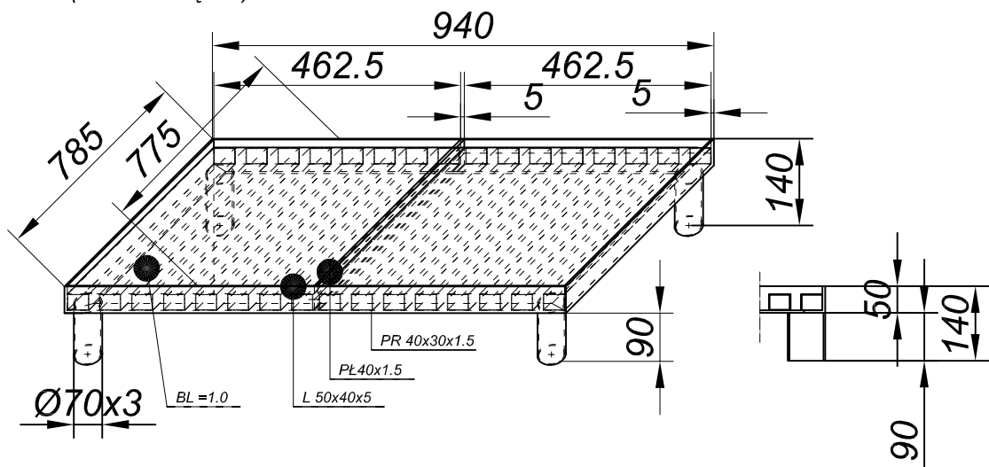
No.4 PALETA 4 (ażurowa)
