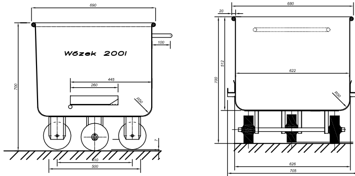
No.99 Wózek farszowy
