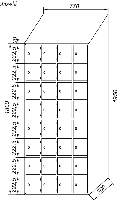
No.76 Schowki
