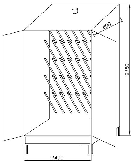
No.89 Suszarka do butów zabudowana
