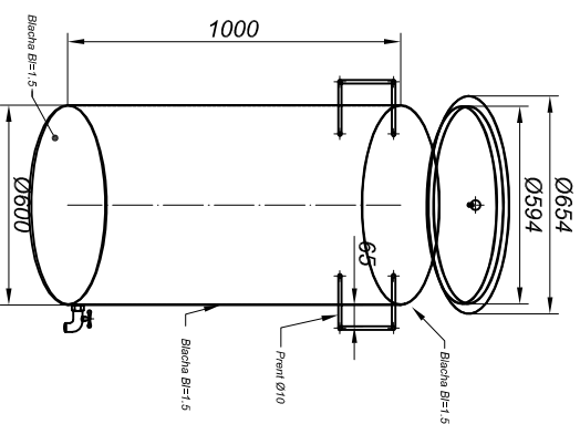
Płaszcz wewnętrzny
