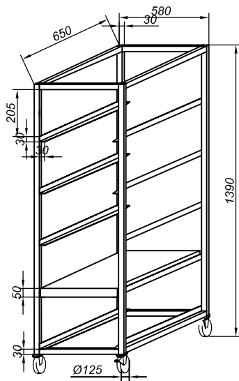
No.94 lada piekarnicza
