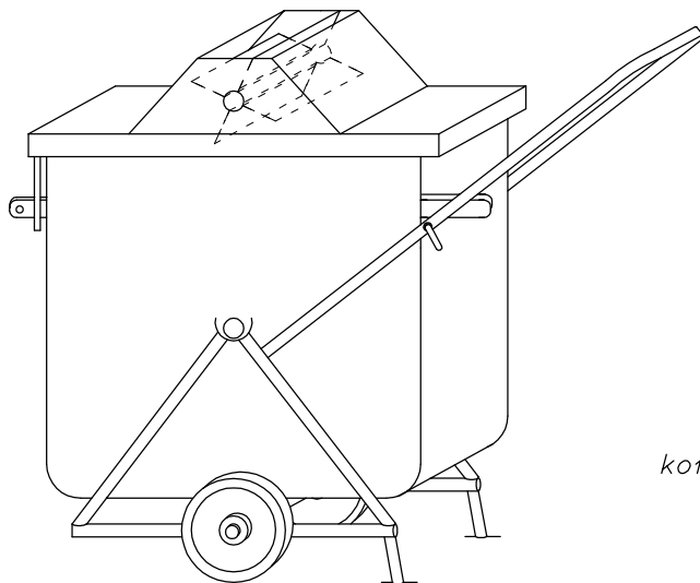
No.107 Konfiskator
