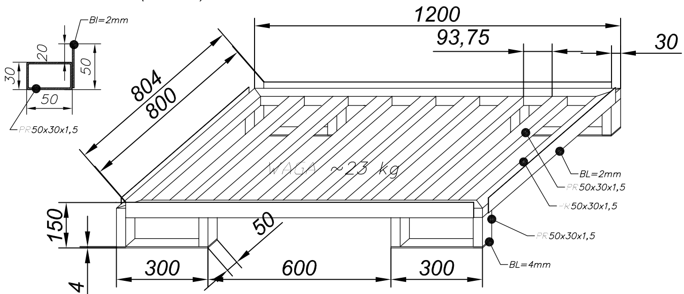
No.4 PALETA 4 (ażurowa)
