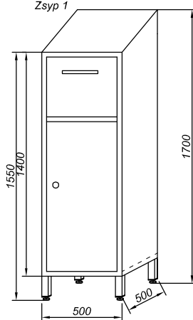
No.73 Zsyp 1
