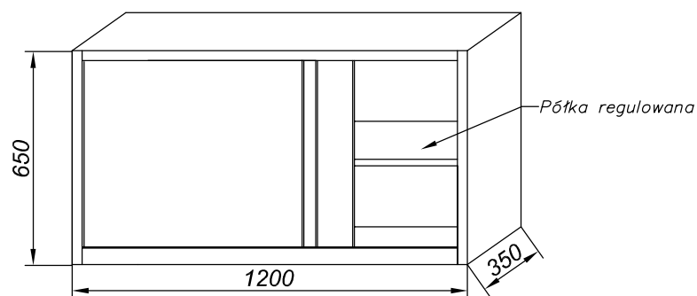
No.58 Szafa w.3
