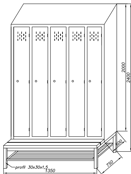
No.68 Szafa 5 z ławką
