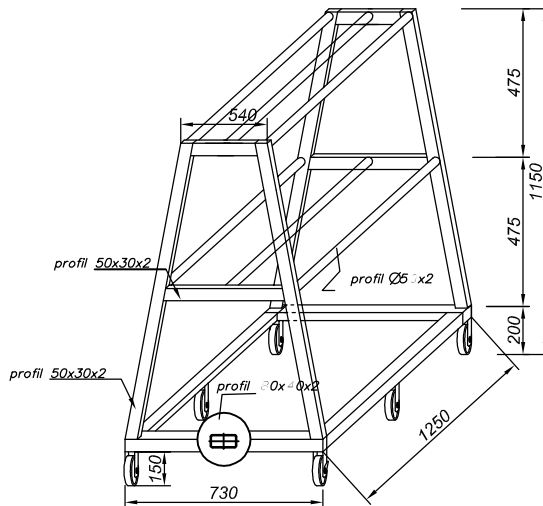
No.98 Wózek
