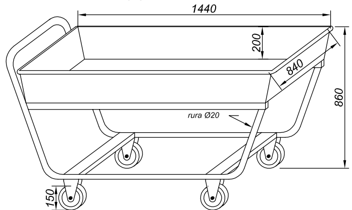
No.104 Wózek
