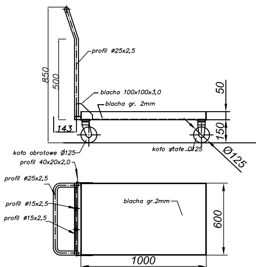
No.102 Wózek transportowy
