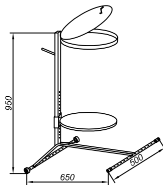
No.91 kosz
