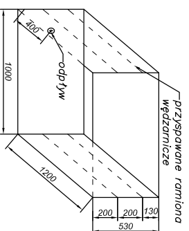
Płaszcz wewnętrzny
