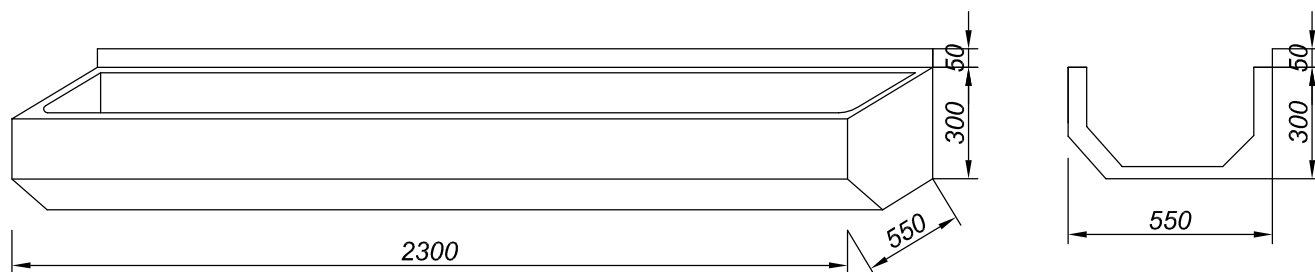
No.51 Rynna wielostanowiskowa
