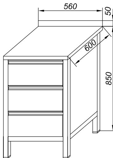
Blok szuflad
