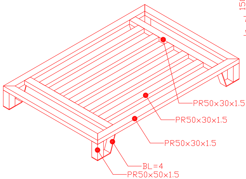
No.80 PALETA 6 (ażurowa)
