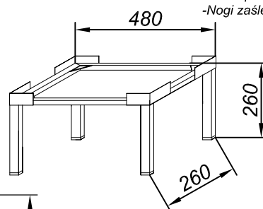
No.23 Podstawa maszyny 2
