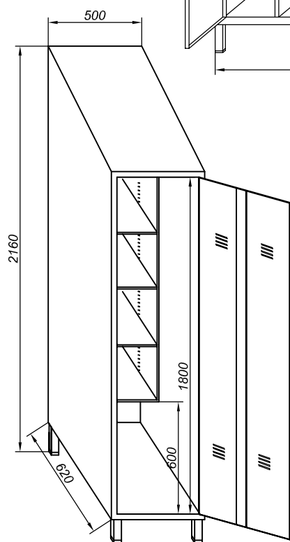
No.74 Szafa na szczotki -Ze skośnym dachem -Zamykanie T-gryfem
