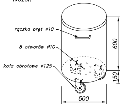
No.105 Wózek
