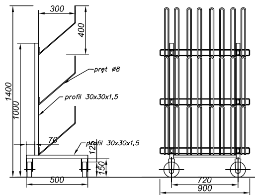
No.99 Wózek
