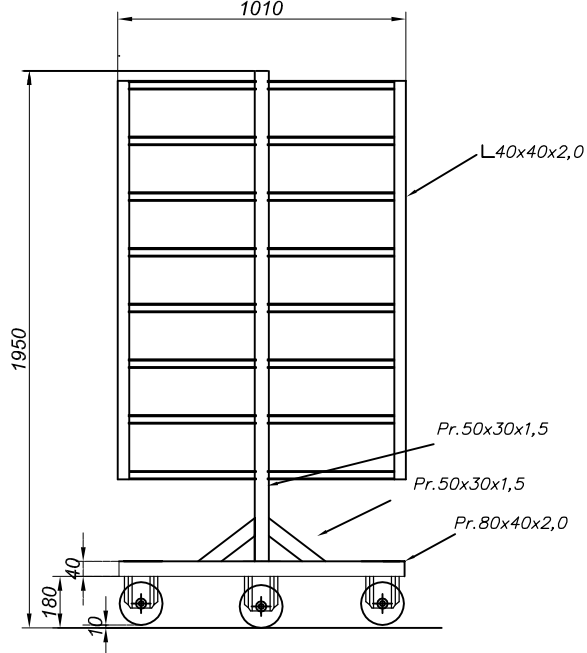
No.109 Wózek wędzarniczy H 1010
