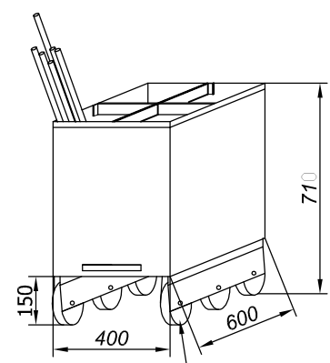
No.102 Wózek do transportu kiji wędzarniczych
