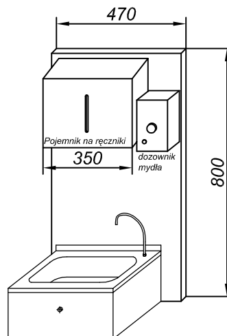
No.82 Panel mały
