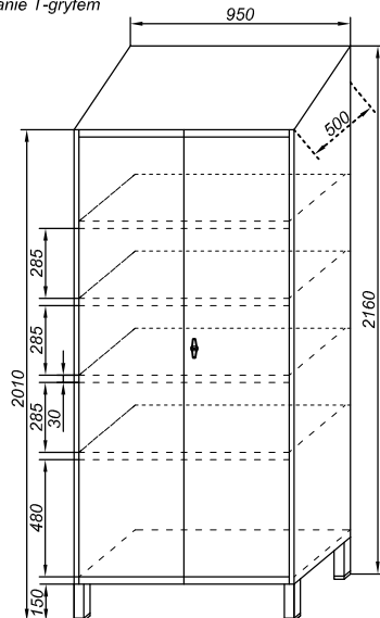
No.72 Szafa wysoka -Ze skośnym dachem -Zamykanie T-grytem
