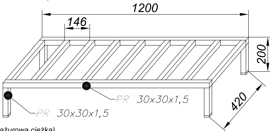
No.3 PALETA 3 (ażurowa ciężka)
