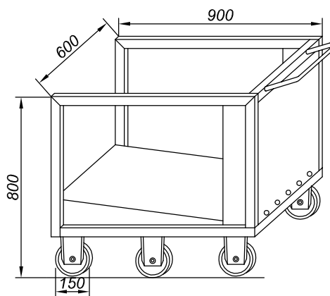
Wózek na kije
