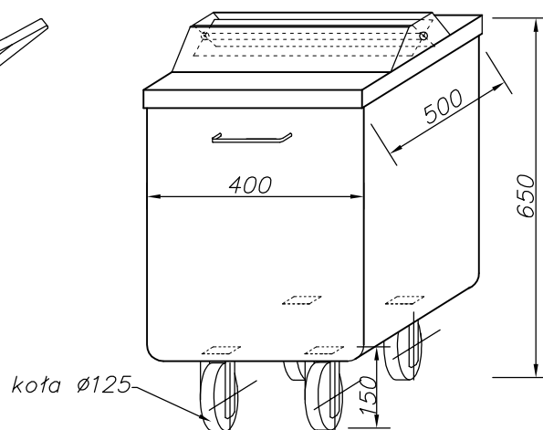
No.108 Konfiskator mały
