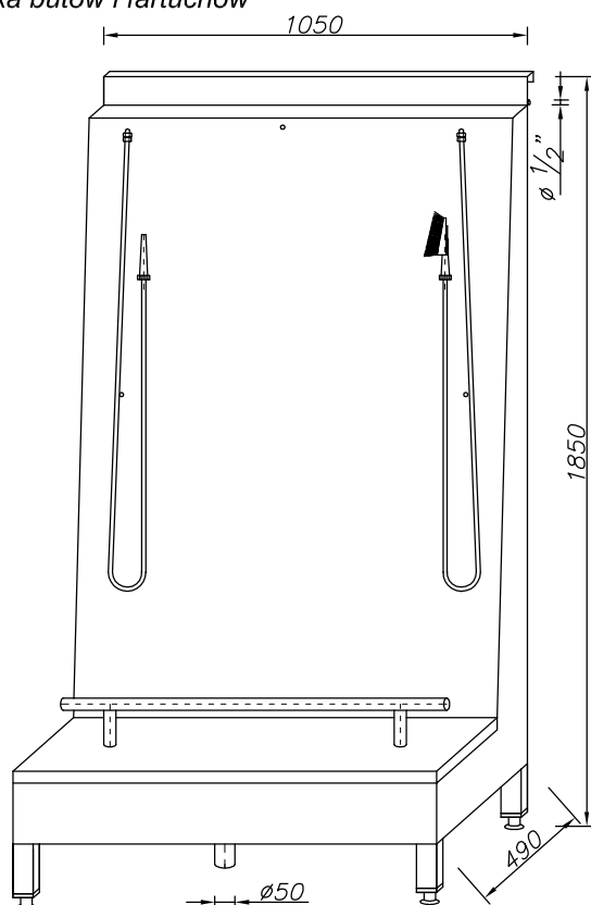
No.86 Myjka butów i fartuchów
