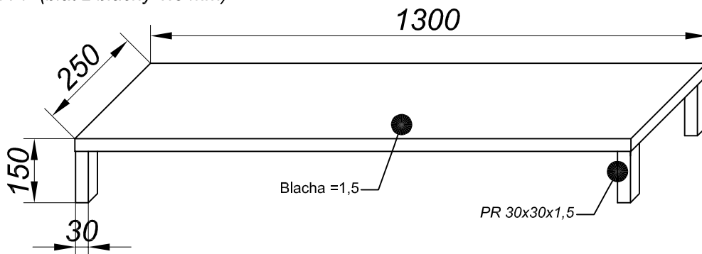
No.2 PALETA 2 (ażurowa lekka)
