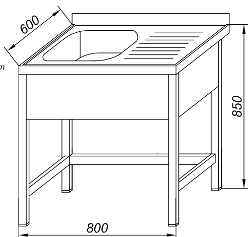
No.40 Zlewozmywak 1
