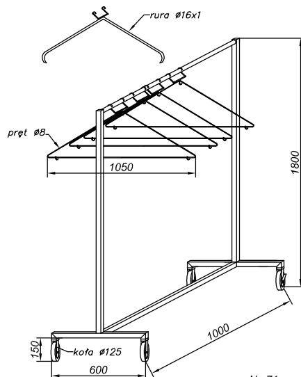
No.71 Wieszak fartuchów 1
