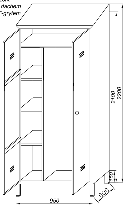
No.77 Szafa
