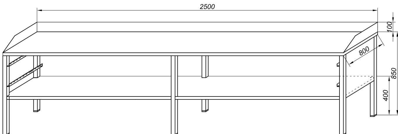
No.21 Stół piekarniczy 1
