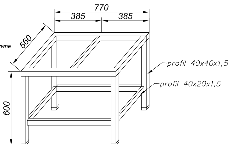
No.23 Podstawa maszyny 2
