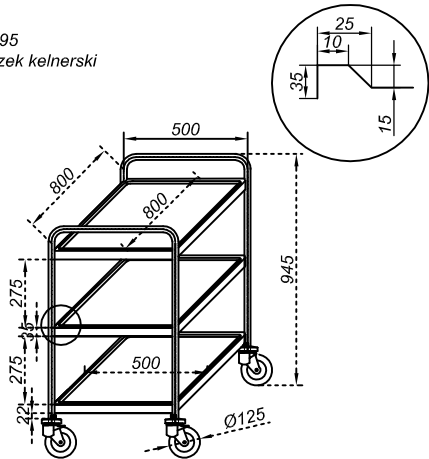
No.97 Wózek kelnerski
