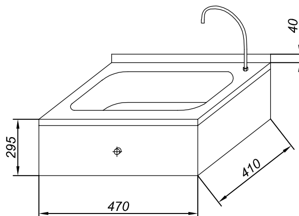
No.53 Zlewozmywak z włącznikiem kolanowym
