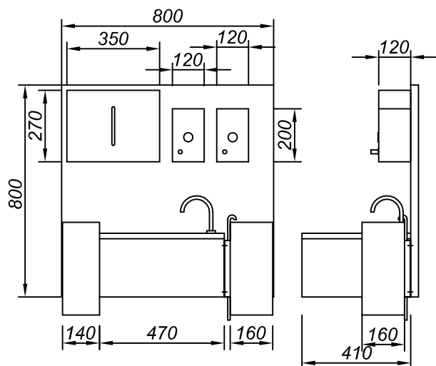
No.81 Panel higieniczny
